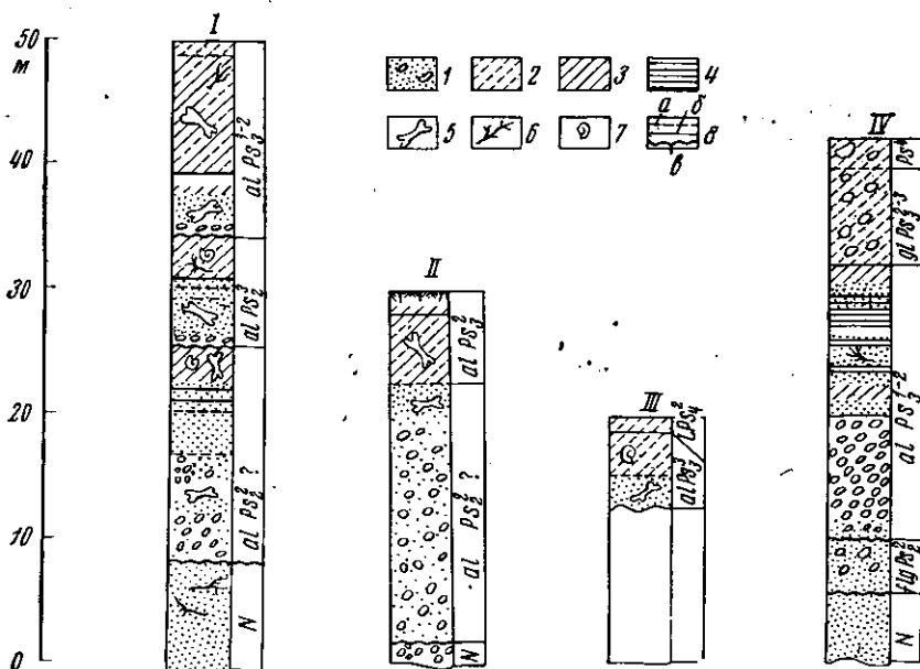
Рис. 2. Схематические стратиграфические колонки по террасам рек Алдана и Тумары
