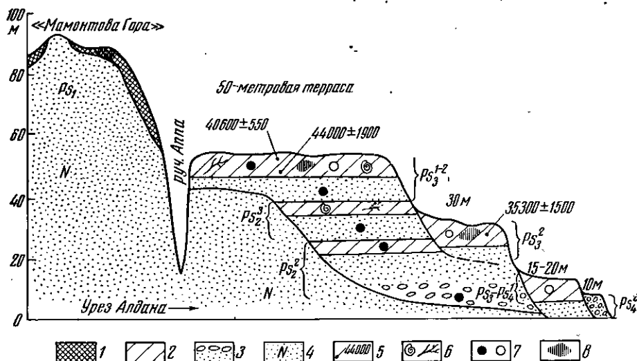
Рис. 1. Схема строения разреза «Мамонтова Гора».
