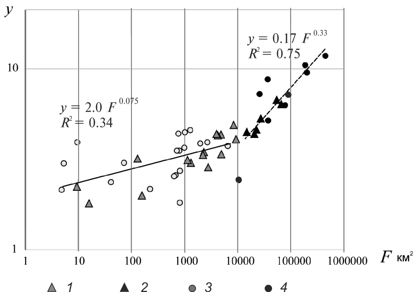
Рис. 2. Зависимость показателя внутригодовой неравномерности стока от площади водосбора Водосборы бассейнов рек Большеземельской тундры площадью, км²: 1 – \leq 10000 , 2 – > 10000 . Водосборы рек бассейна р. Вилюй площадью, км²: 3 – \leq 10000 , 4 – > 10000
