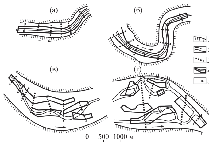
Рис. 3. Оконтурирование блоков подсчета запасов золота на участках долин с относительно прямолинейным неразветвленным руслом (а), с развитием врезанных излучин (б), свободных излучин (в) и русла, разветвленного на рукава (г).
