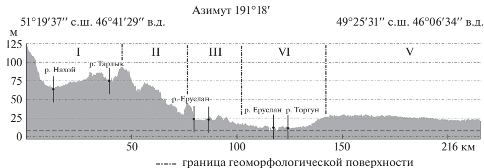
Рис. 2. Профиль рельефа 124-20, пересекающий геоморфологические поверхности мезозектона “Малый Сырт”.
