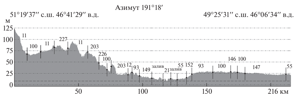
Рис. 6. Профиль 124-20 с приуроченными границами контуров почв.
