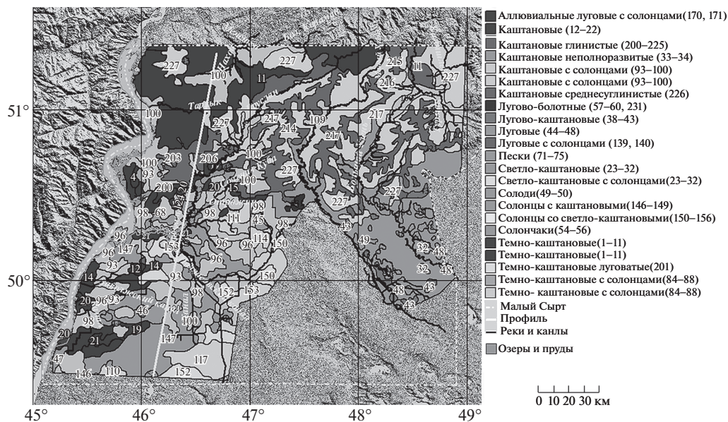
Рис. 5. Почвенная схема мезозкотона "Малый сырт".
