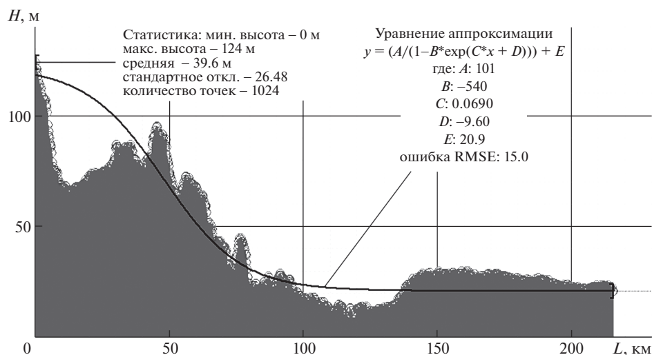
Рис. 3. Модель профиля рельефа 124-20 мезозектона “Малый Сырт”.
