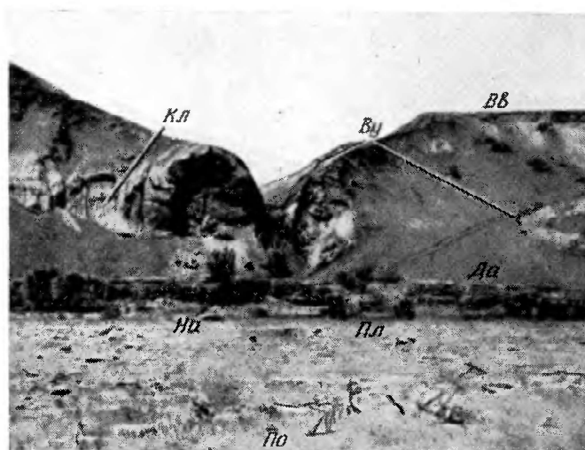
Рис. 2. Западное побережье Аральского моря к югу от м. Актумсык
