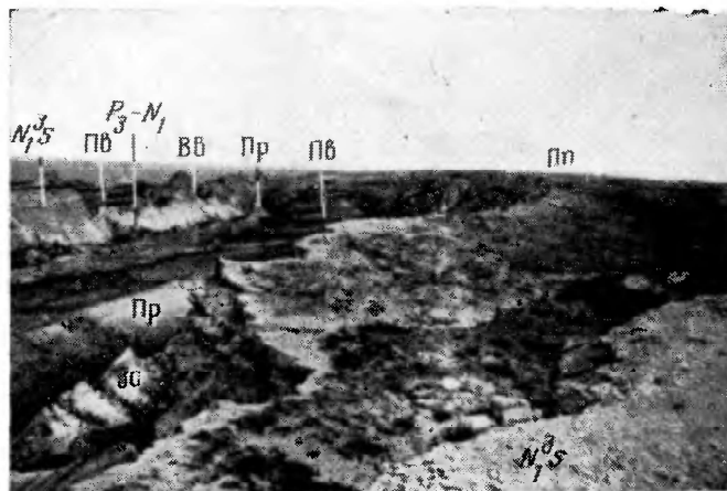
Рис. 3. Восточный чинк Устюрта и промежуточная ступень в районе м. Улькентумсык
