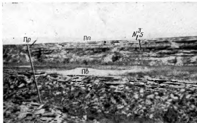
Рис. 4. Восточный чинк Устюрта и продольная впадина севернее урочища Кабанбай Усл. обозн. см. рис. 1
