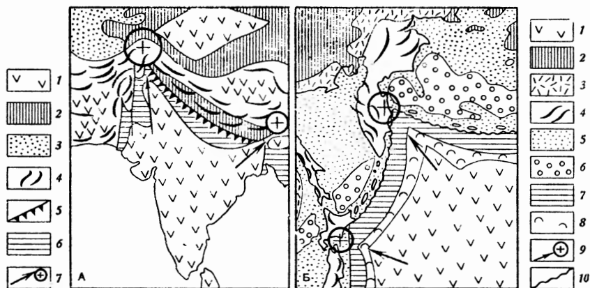
Рис. 1. Основные морфоструктуры внутриконтинентальной (А) и континентально-океанической (Б) шовных зон
