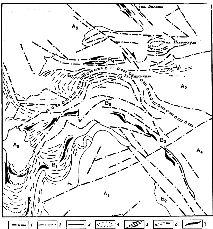
Рис. 2. Основные морфоструктурные элементы внутриконтинентальной шовной зоны
