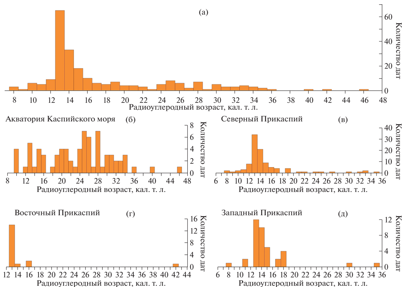
Рис. 4. Радиоуглеродные даты хвалыньских отложений.
