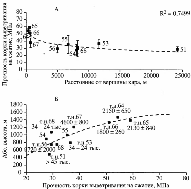
Рис. 5. Связь прочности выветрелой корки ледниковых валунов с их расстоянием от области питания (А) и абсолютной высотой (Б)
