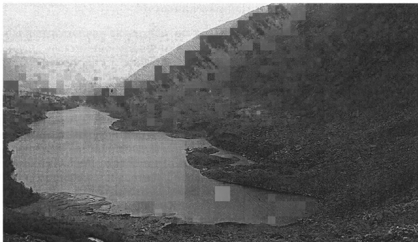
Рис. 3. Активный присклоновый лопастной каменный глетчер в истоках руч. Левада. Мандычанский массив (хр. Черского)
