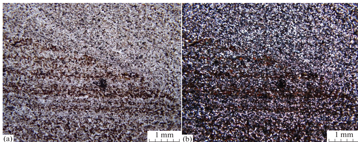
Fig. 6. Thin section SA19 – 242.1 cm. The oblique texture of the silty layers of the CMSfs lithotype. (a) – PPL, (b) – XPL. Рис. 6. Шлиф SA19 – 242.1 см. Косая текстура алевритовых слоев в литотипе CMSfs. (a) – PPL, (b) – XPL.
