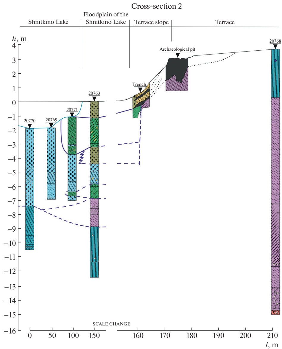
Fig. 5. Toropa river valley cross-section 2. See fig. 4 for legend. Рис. 5. Геолого-геоморфологический профиль 2 через долину р. Торопа. Усл. обозначения см. рис. 4.
