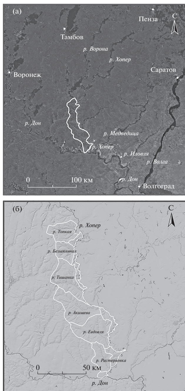
Рис. 2. Картограммы расположения и структуры водосборов объекта исследований: (а) – расположение объекта, (б) – структура водосборов объекта.
