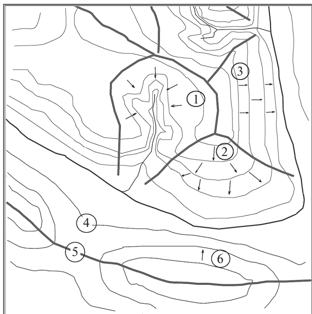
Рис. 1. Картограмма склонов различных типов. Склон: 1 – собирающий (водосбор), 2 – рассеивающий (межводосборный участок склонов), 3 – нейтральный (межводосборный участок склонов); 4 – изолиния рельефа; 5 – линия водораздела; 6 – линия стока поверхностных вод.
