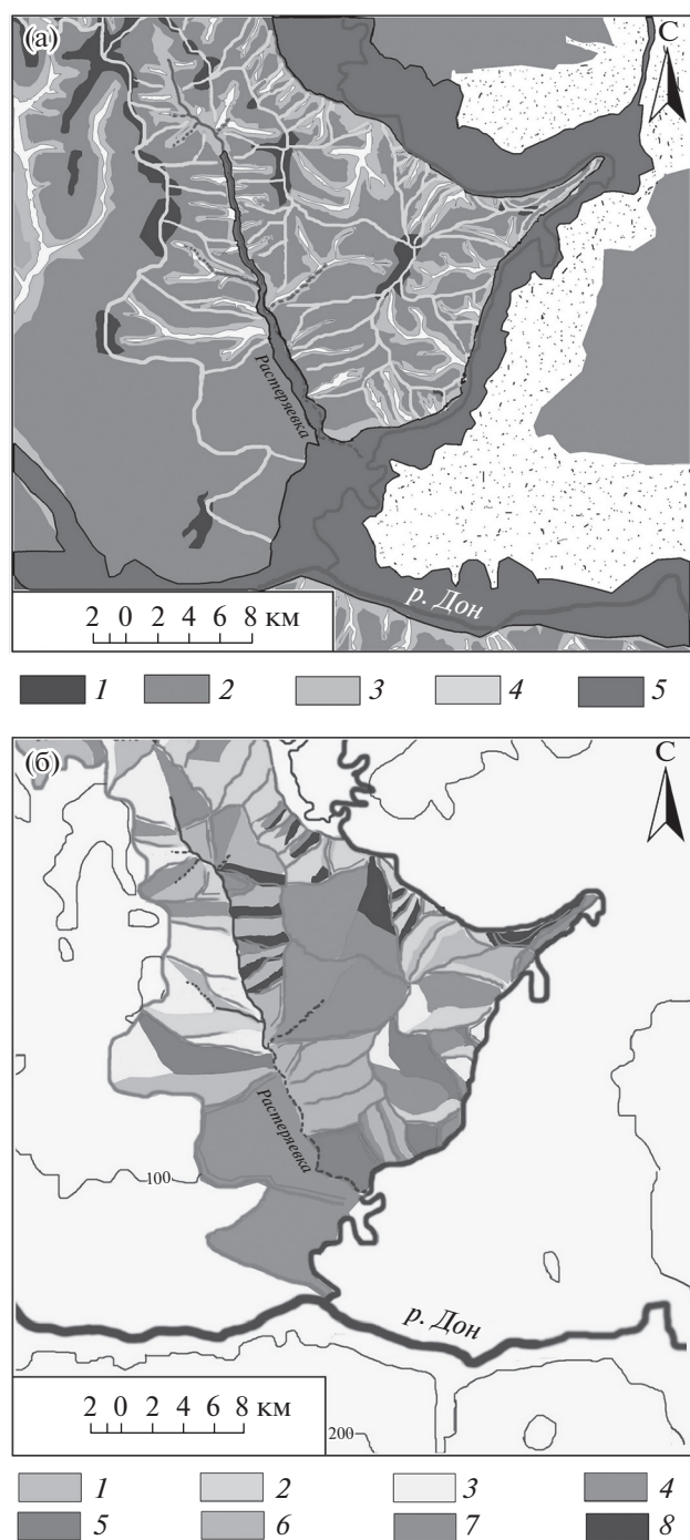
Рис. 8. Фрагменты карт правобережья р. Хопер: (а) — крутизна склонов водосборов и участие речных долин, (б) — экспозиция склонов водосборов. (а) — крутизна склонов : 1 — 0–0.5°; 2 — 0.6–3°; 3 — 4–7°; 4 — 8–35°; 5 — речные долины. (б) — экспозиция склонов : 1 — северная, 2 — северо-восточная, 3 — восточная, 4 — юго-восточная, 5 — южная, 6 — юго-западная, 7 — западная, 8 — северо-западная.
