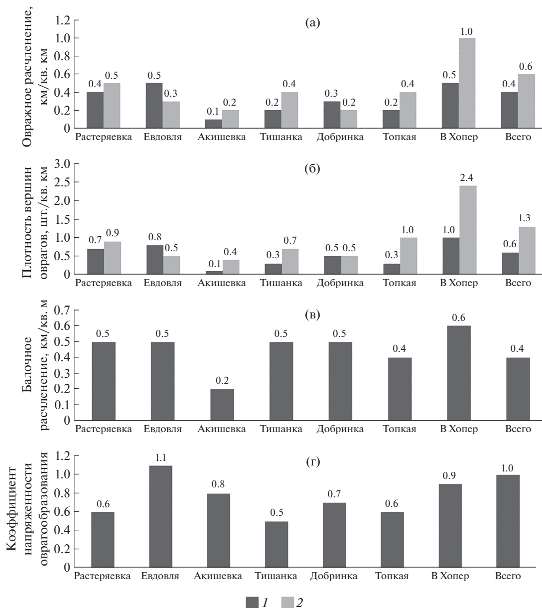
Рис. 5. Среднеарифметические показатели эрозионного состояния собирающих водосборов и междовосборных участков склонов: (а) – овражного расчленения, (б) – плотности вершин оврагов, (в) – балочного расчленения, (г) – коэффициента напряженности оврагообразования (отношение овражного расчленения к древнему (балочному)). 1 – собирающие водосборы, 2 – междовосборные участки склонов.
