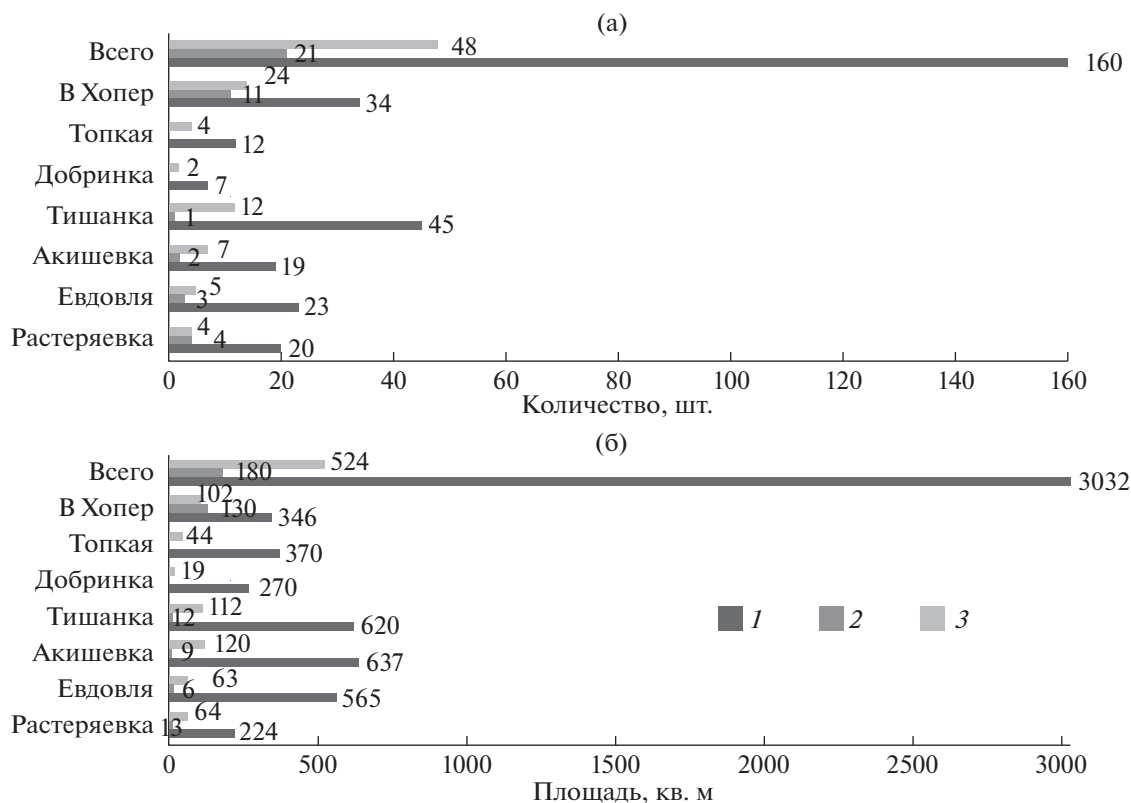
Рис. 3. Структура водосборов правобережья р. Хопер: (а) — количество собирающих водосборов и междоводосборных участков склонов, (б) — занимаемая площадь собирающими водосборами и междоводосборными участками склонов. 1 — собирающие водосборы; склоны (междоводосборные участки склонов): 2 — прямые, 3 — рассеивающие.
