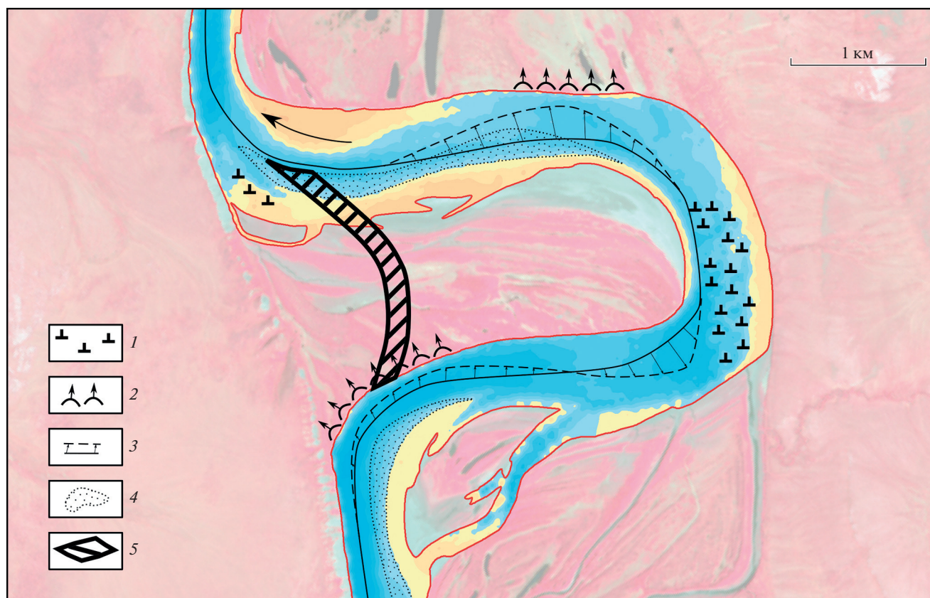
Рис. 4. Прогнозная оценка переформирования русла: 1 — скальные выходы в потоке; 2 — развитие вогнутости размываемого берега, оказывающее направляющее воздействие на поток; 3 — изменение положения динамической оси потока; 4 — зоны аккумуляции наносов; 5 — гидравлически оптимальное положение оси потока при спрямлении излучины и рекомендуемая прорезь-канал через шпору излучины.
